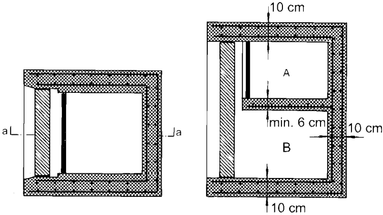
vue en coupe a-a
