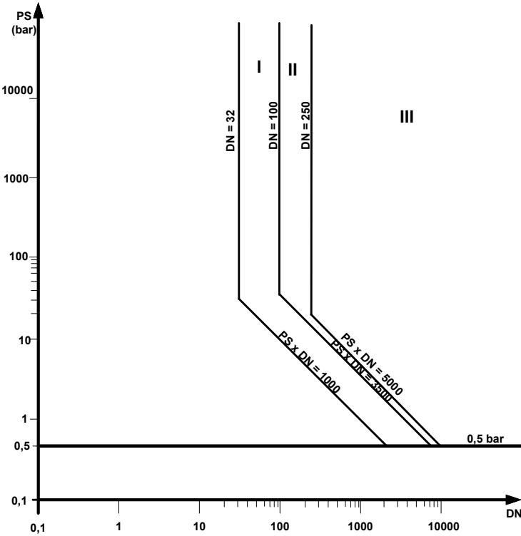
Diagramm 7 für Rohrleitungen nach Artikel 5 Absatz 2 Buchstabe d Ziffer 2
