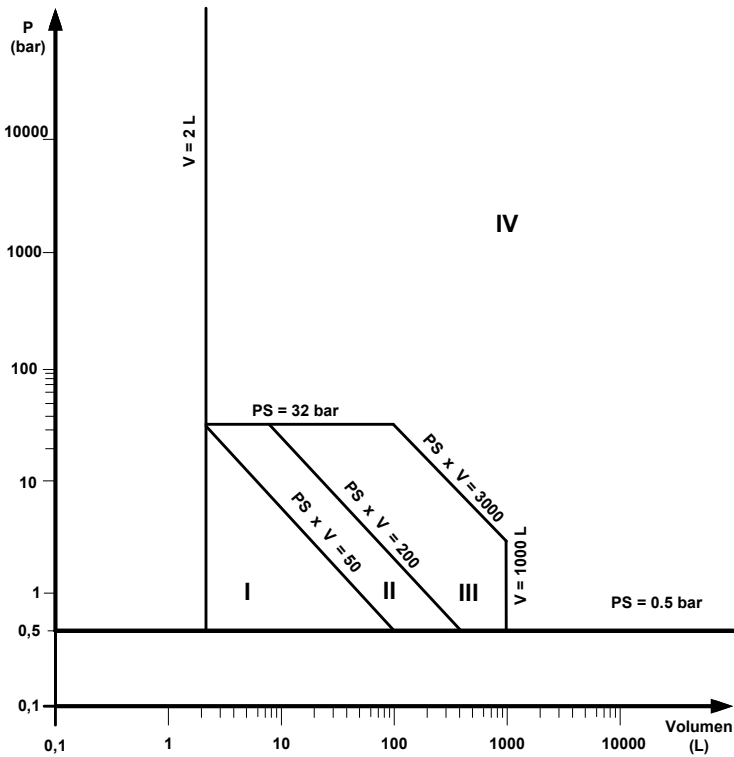
Diagramm 5 für Druckgeräte nach Artikel 5 Absatz 2 Buchstaben c und h
